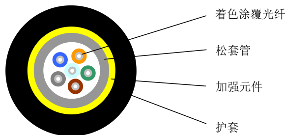
松套管结构引入光缆 I 型
